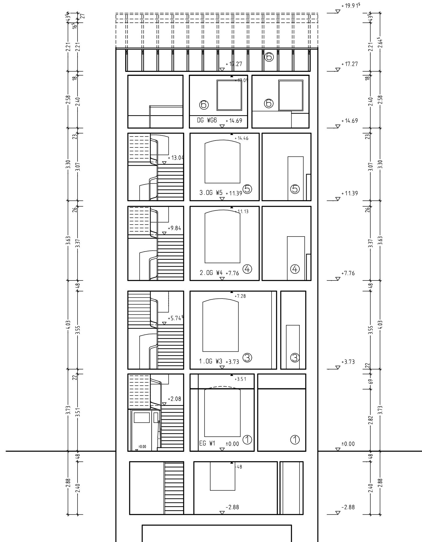
Schnitt A-A Trimbornstraße 11, 51105 Köln
