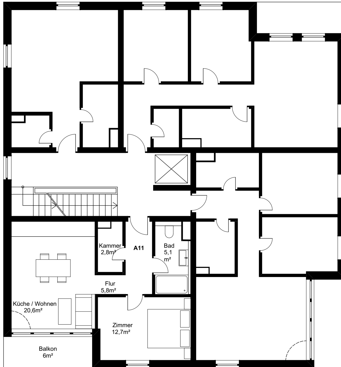
Grundriss 2. Obergeschoss
