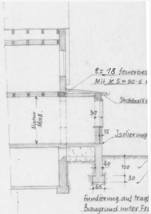
SCHNITT I
