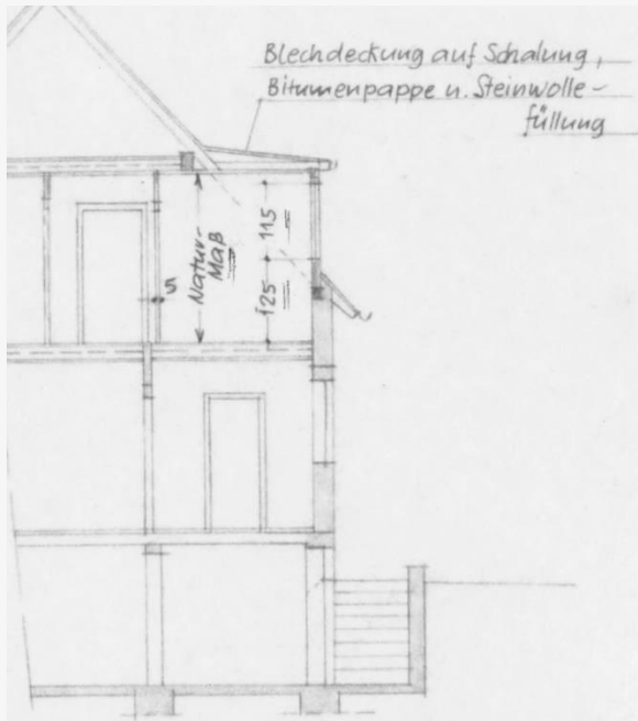
HNITT II
