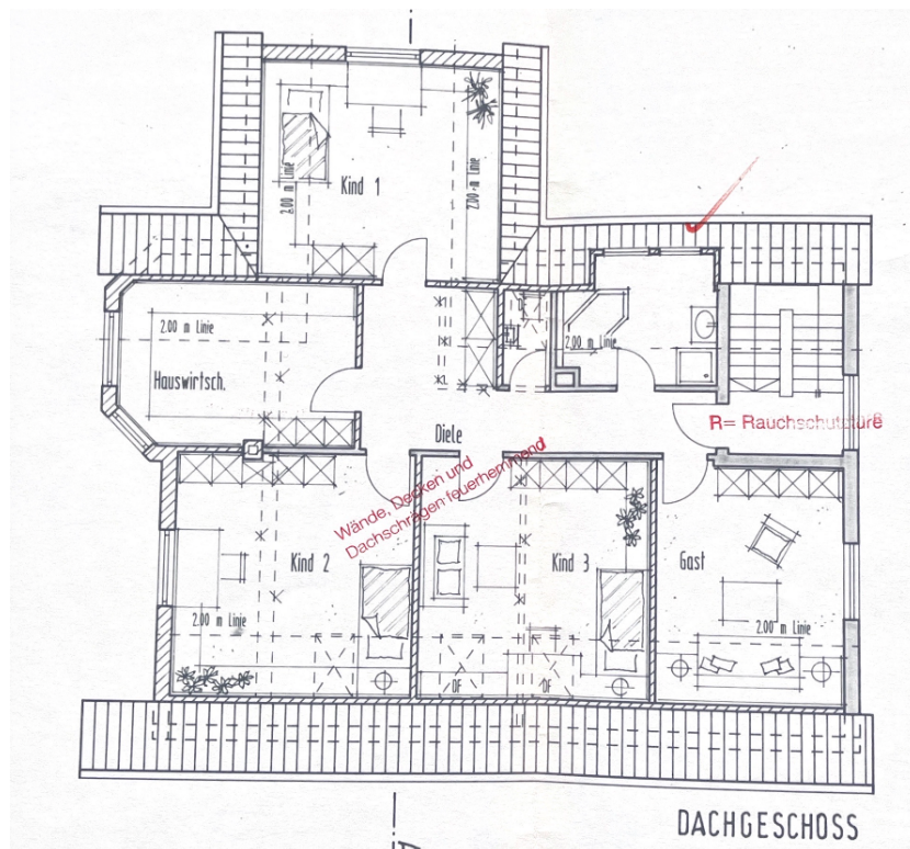
Grundriss Dachgeschoss
