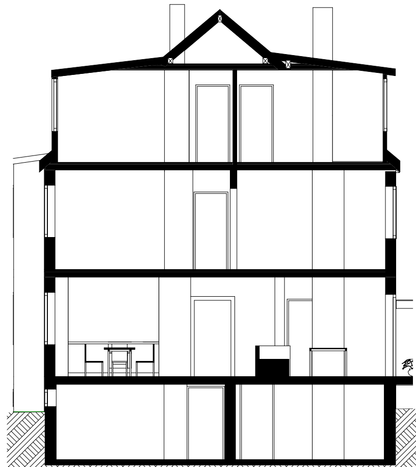
S-A Schnitt A-A 1:100
