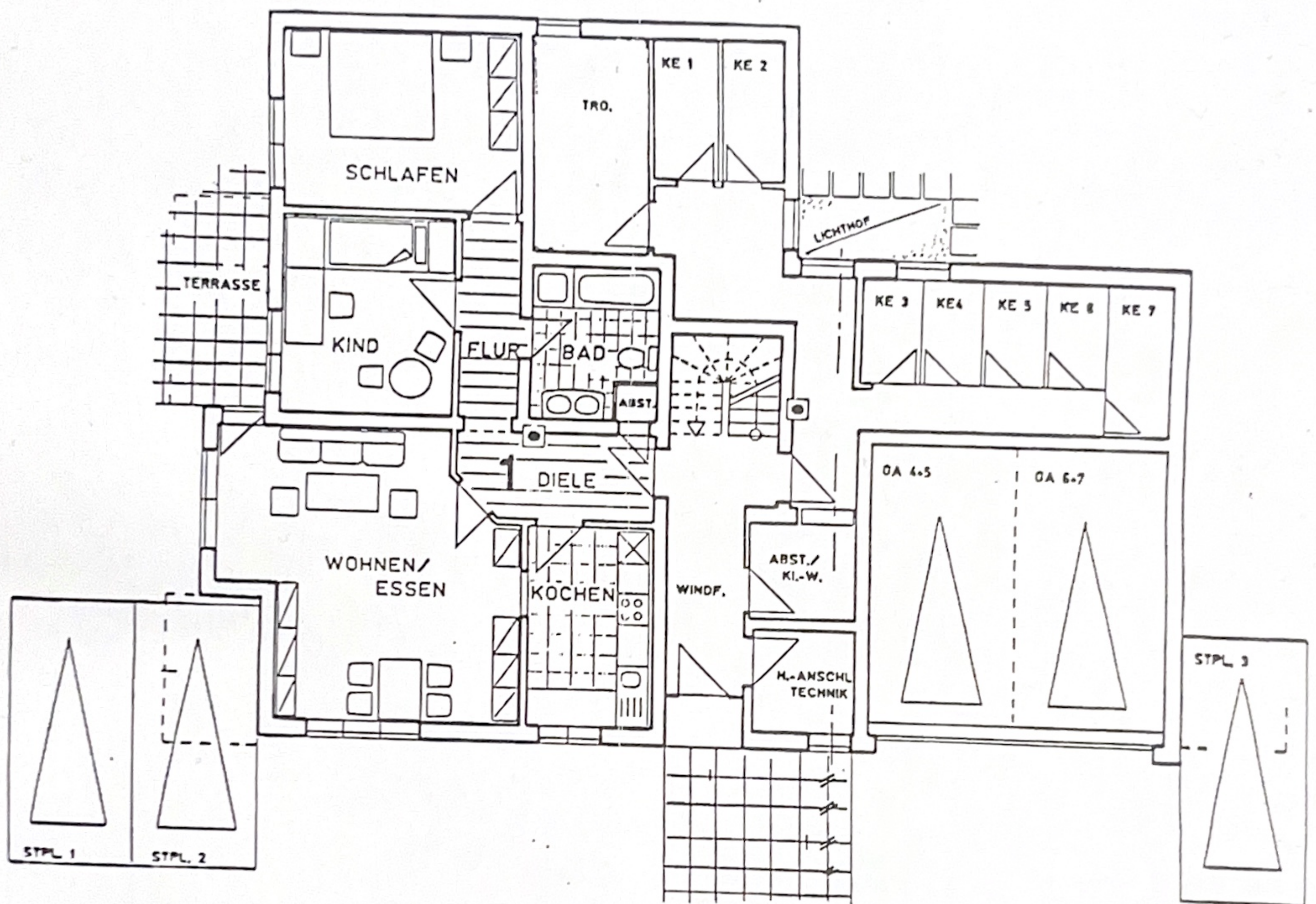
ERDGESCHOSS
