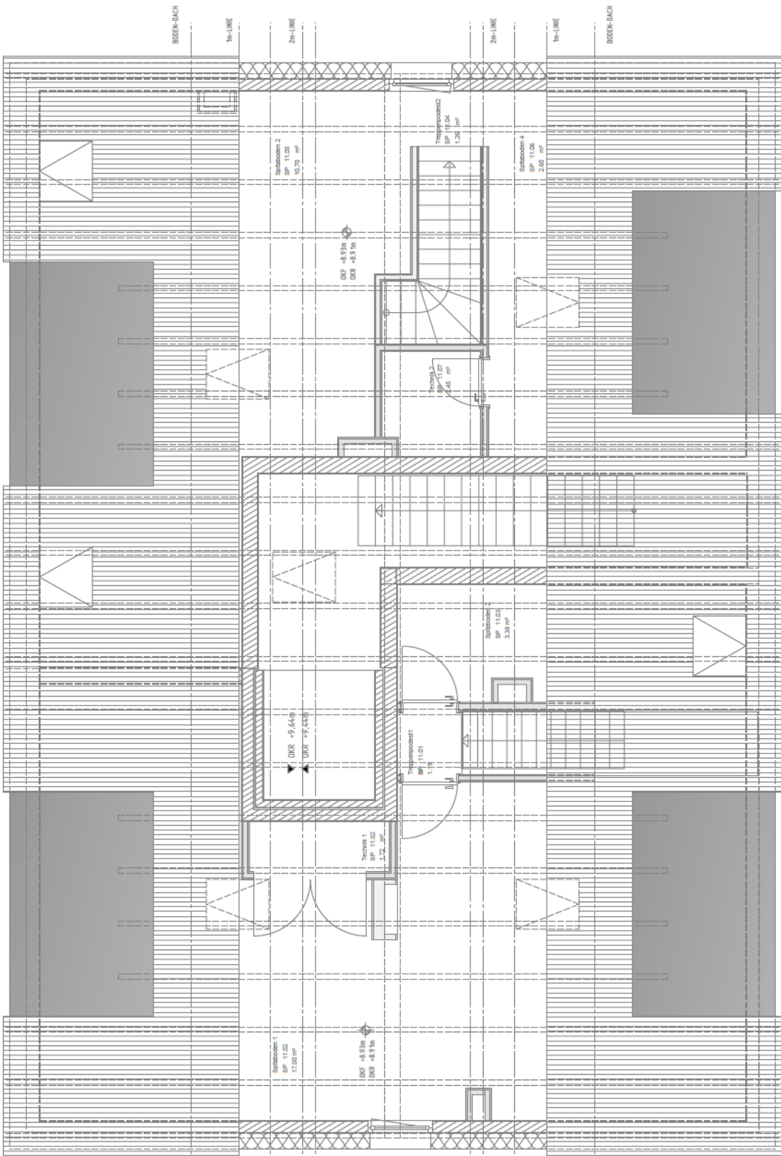
Grundriss Spitzböden
