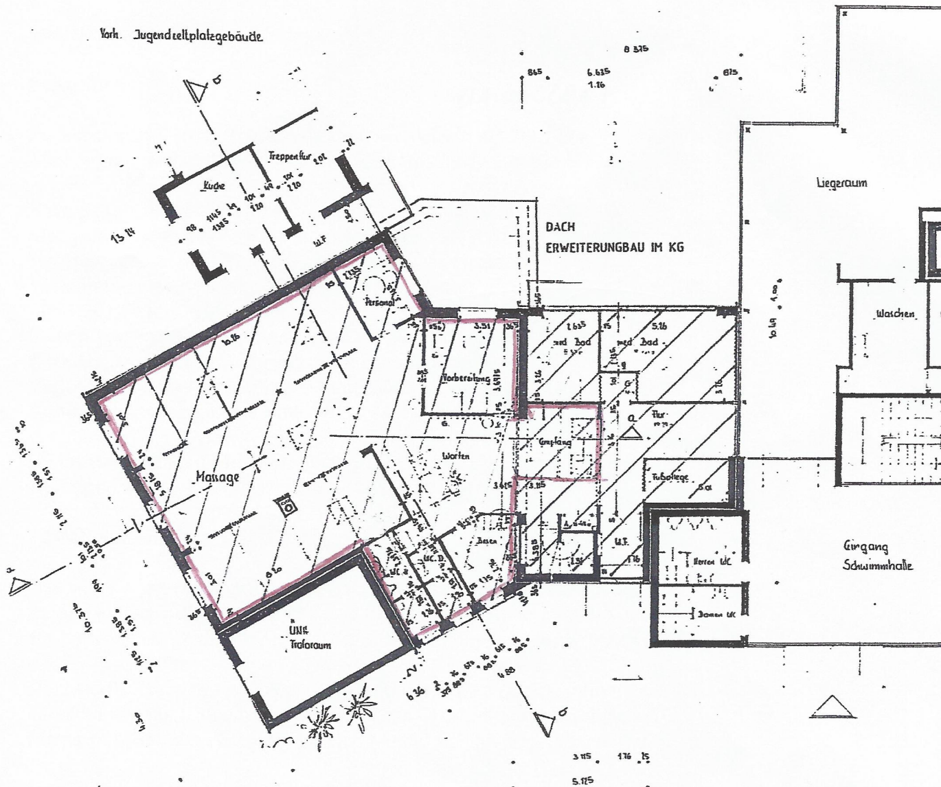
ERDGESCHOSS - GRUNDRISS
