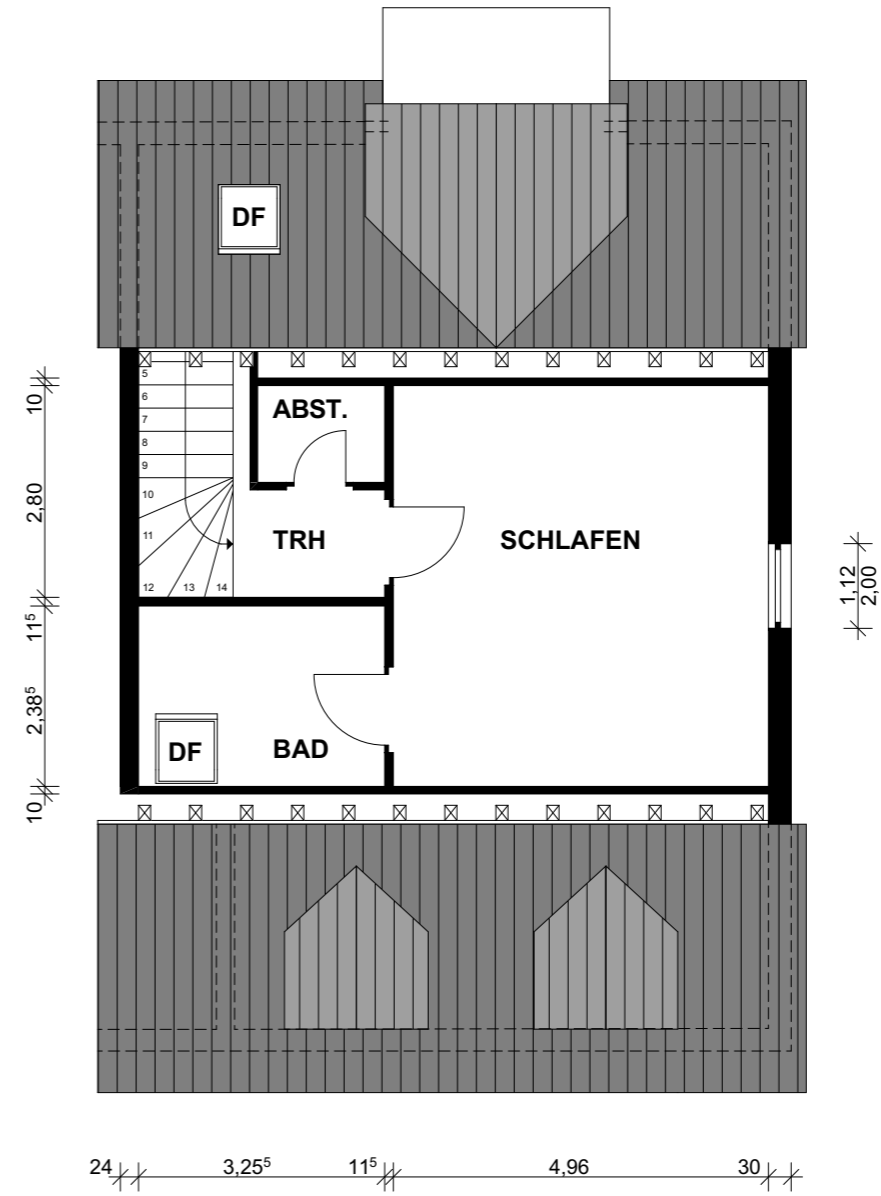
GRUNDRISS EBENE 2
