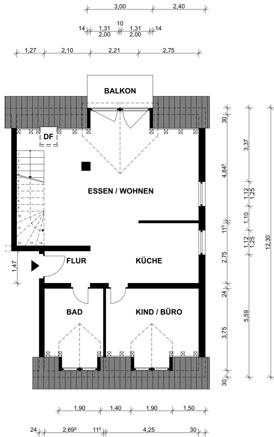
GRUNDRISS EBENE 1
