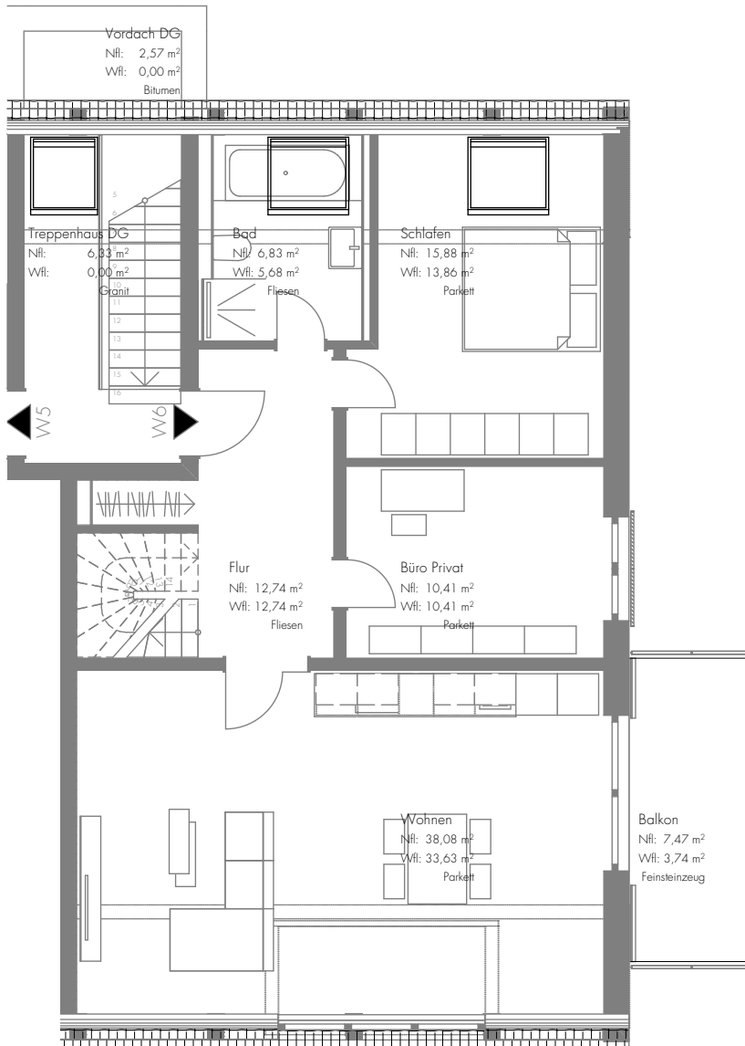
Dachgeschoss
