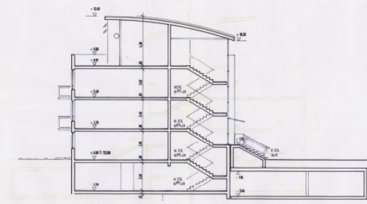
SCHNITT B - B
