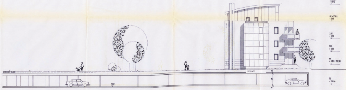
SÜDFASSADE HAUS B
