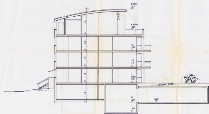
SCHNITT D-D
