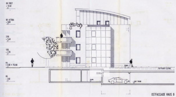
OSTFASSADE HAUS B
