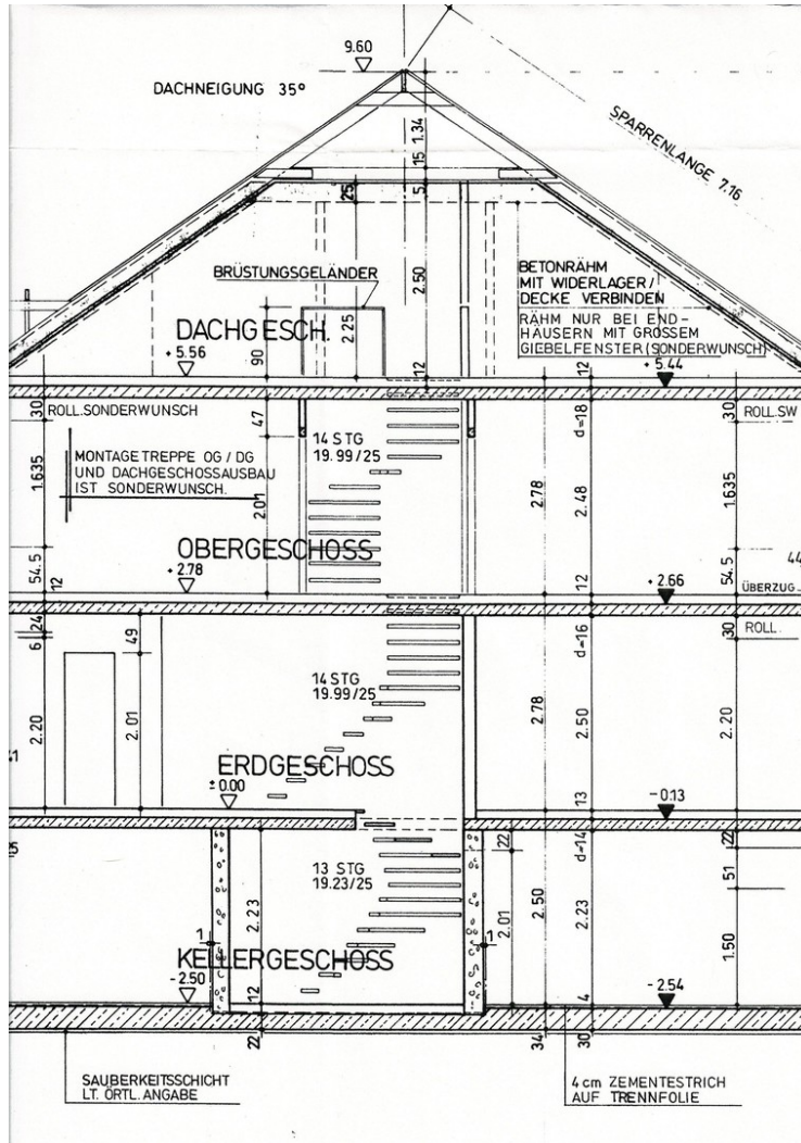
Schnitt Gebäude
