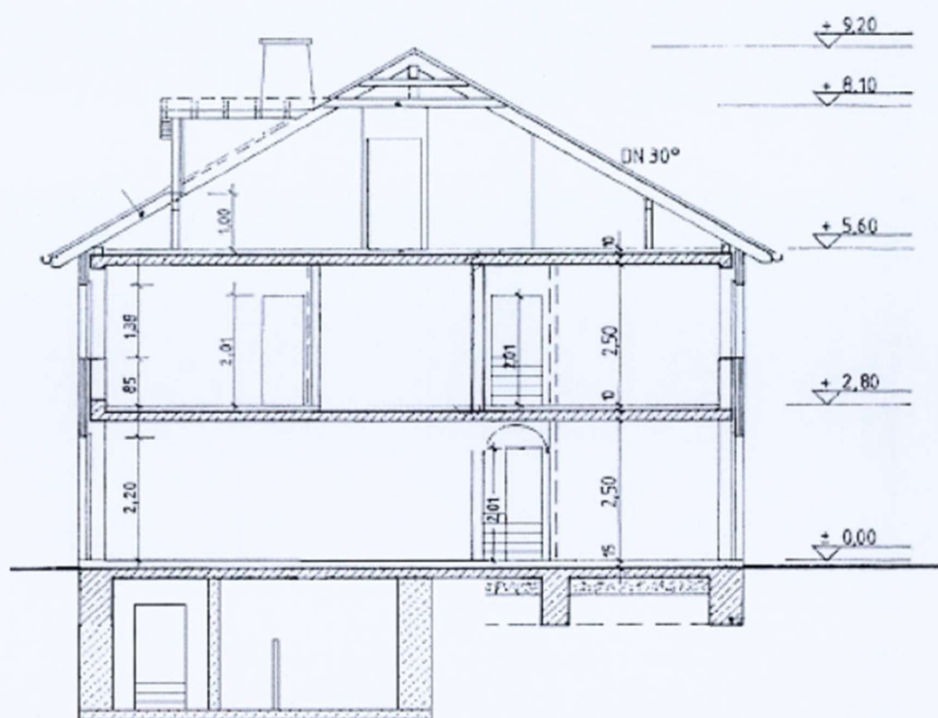
Schnitt M 1:100
