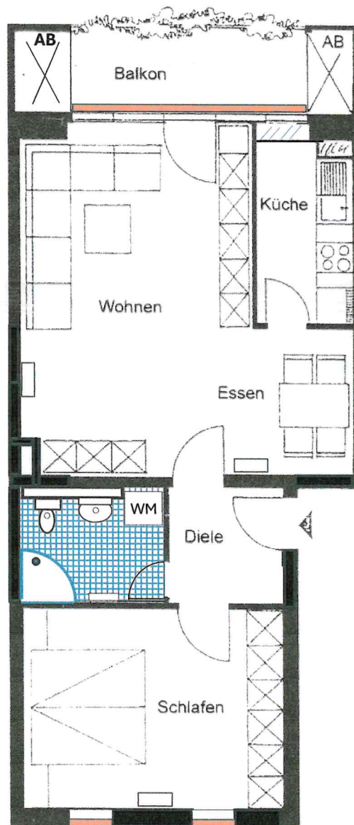
Grundriss
