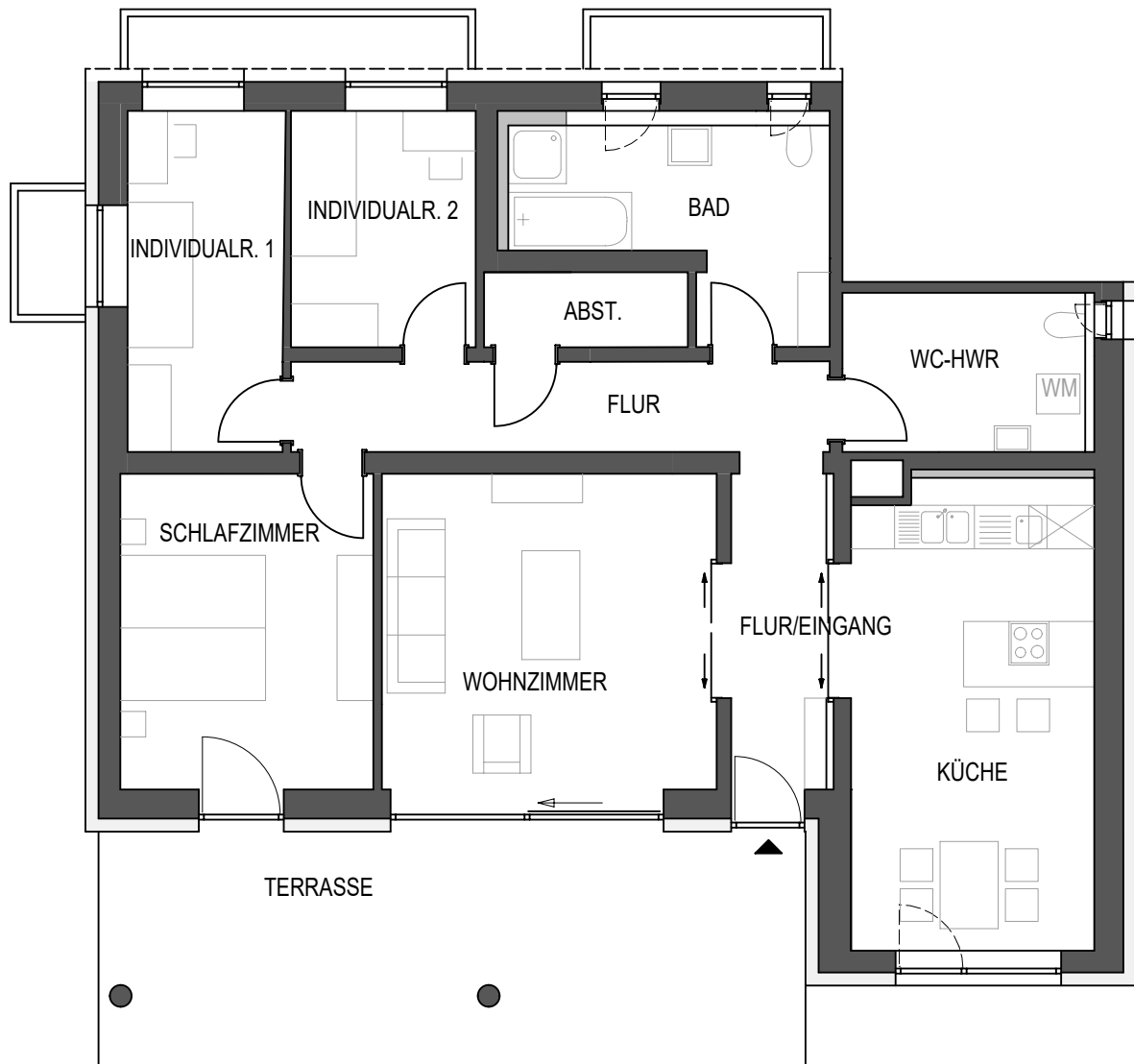
ERDGESCHOSS
