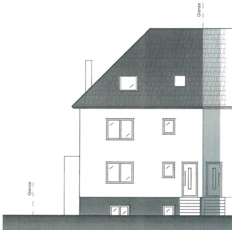
Ansicht Ost
