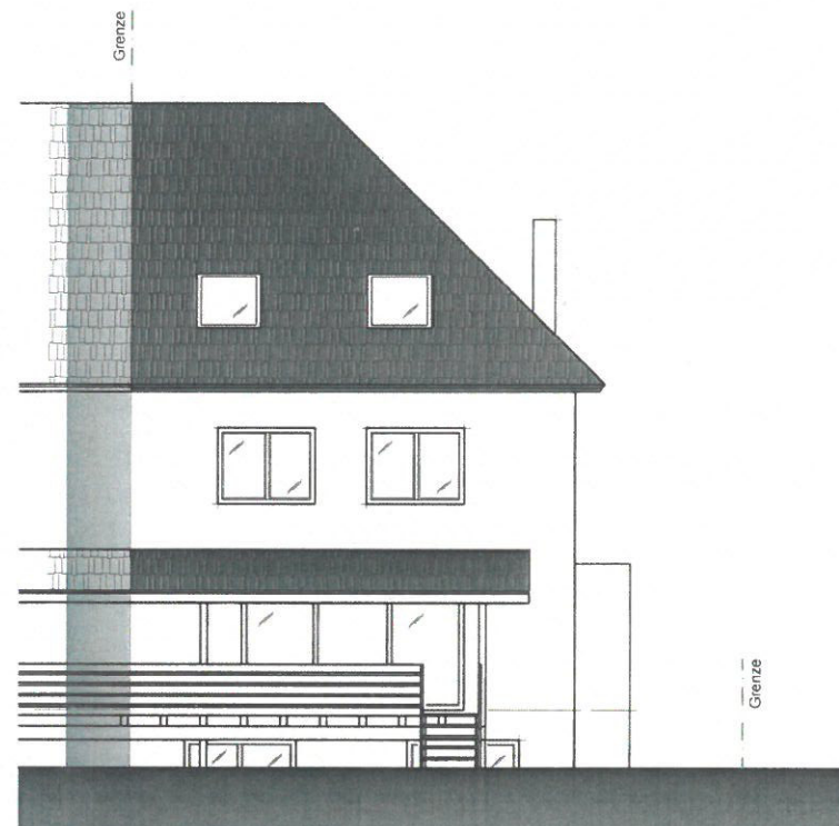
Ansicht West
