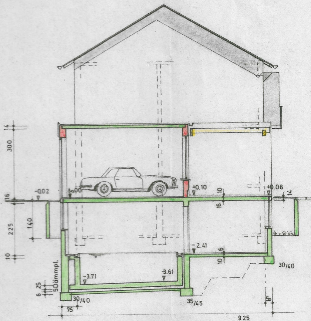
SCHNITT II-II
