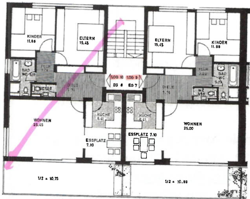
Grundriß Haus A2 Erd- und Obergeschoß
