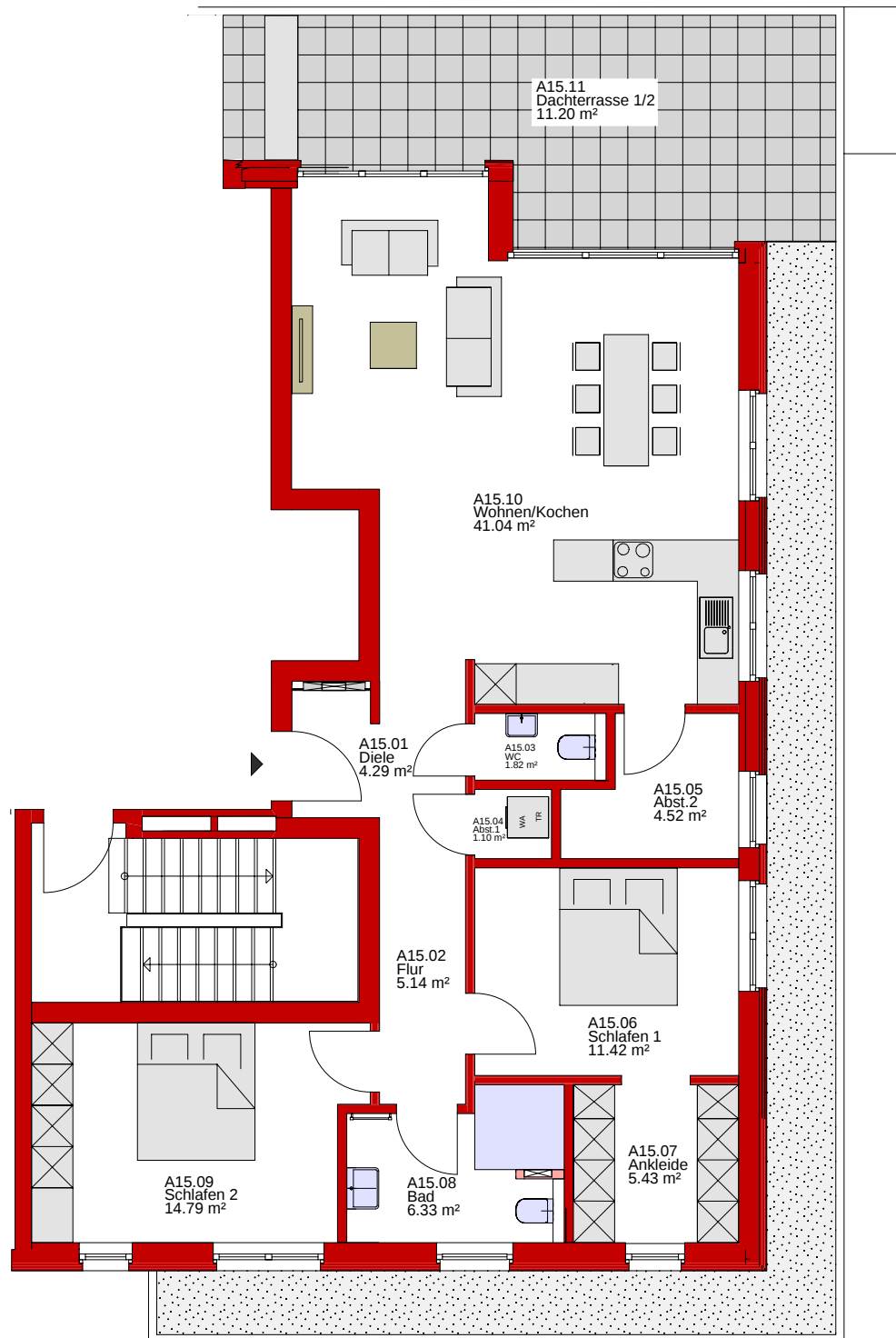
Haus A Staffelgeschoss Wohnung A.15 - 107,22 m 2
