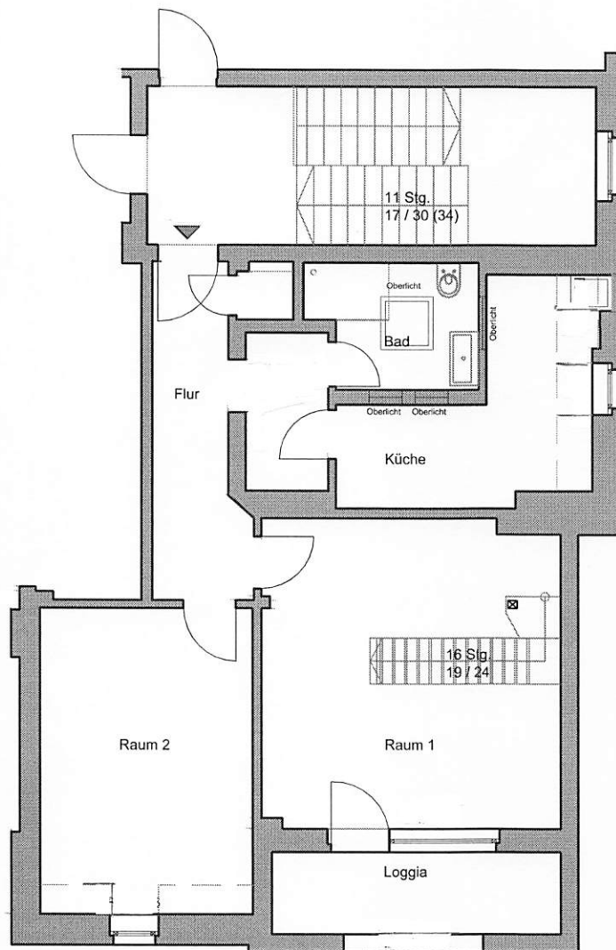
Grundriss Wohnung
