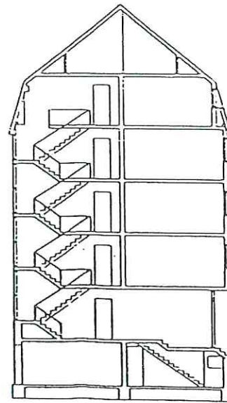
Schnitt a-a
