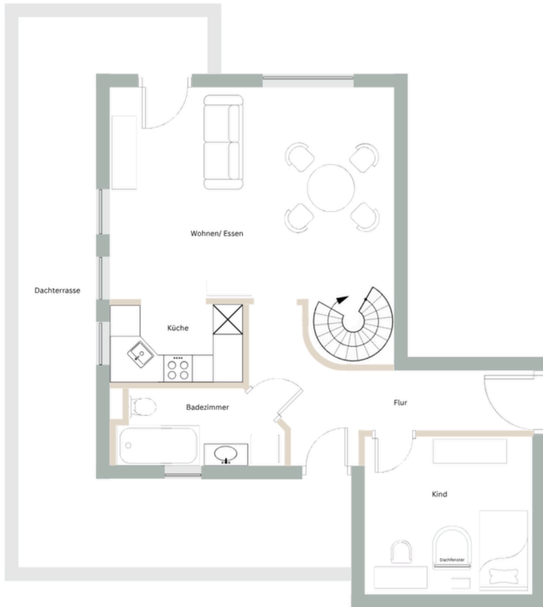
Grundriss 2 Obergeschoss
