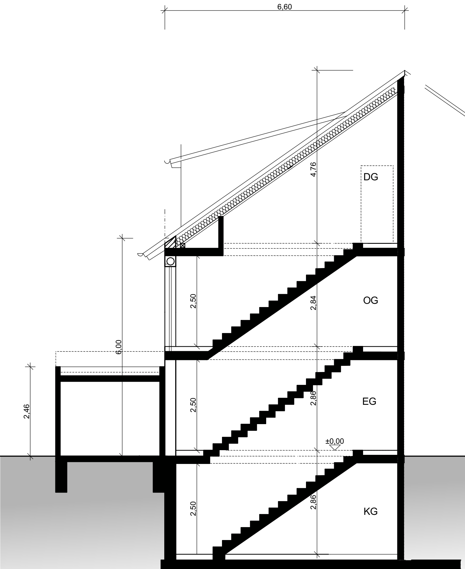
Schnitt A-A
