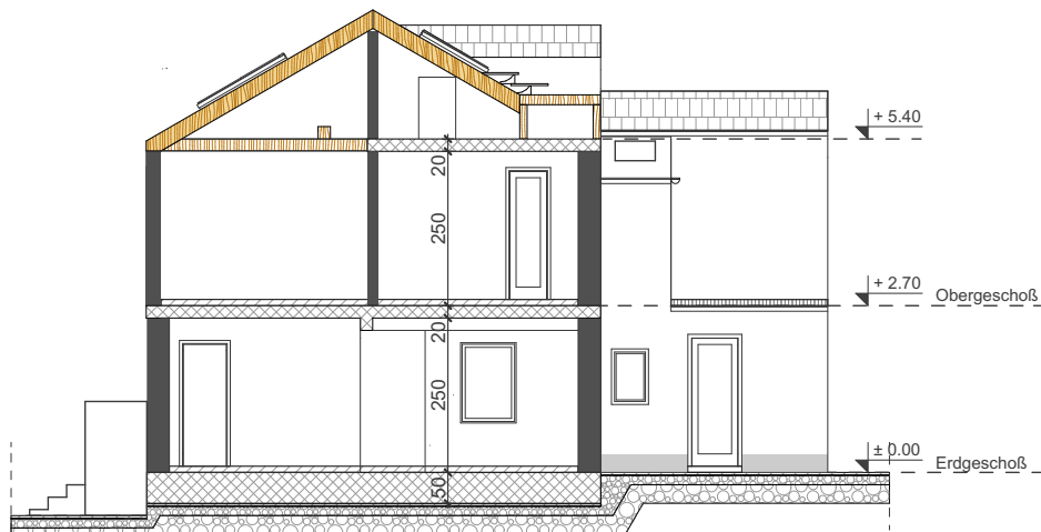
Schnitt 1-1 / Vorderhaus
