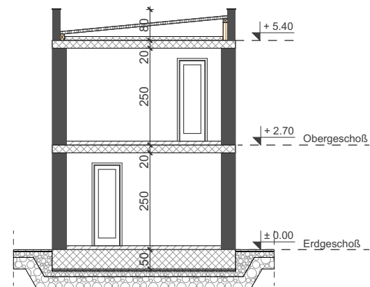
Schnitt 2-2 / Hinterhaus
