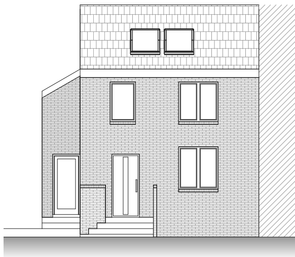
Vorderansicht / Vorderhaus
