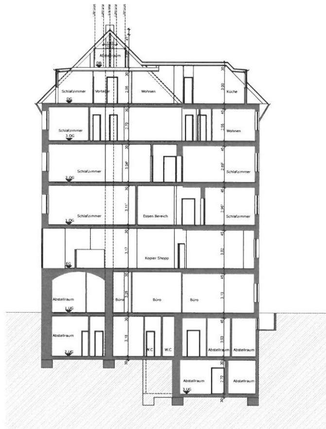
Schnitt A-A
