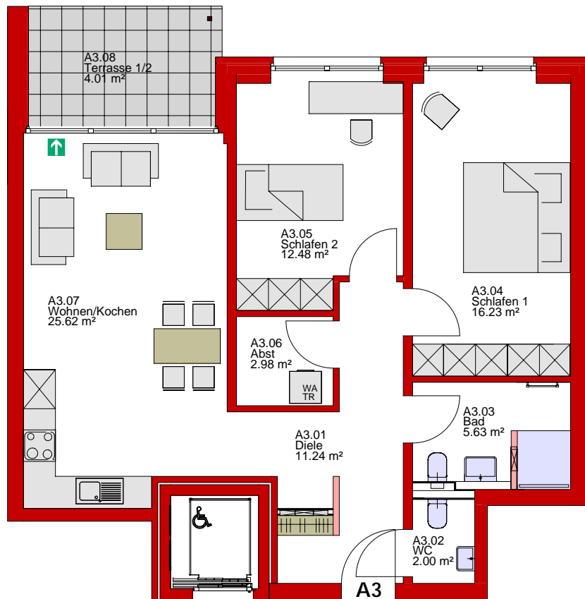
Haus A Erdgeschoß Wohnung A.3 - 79,10 m 2
