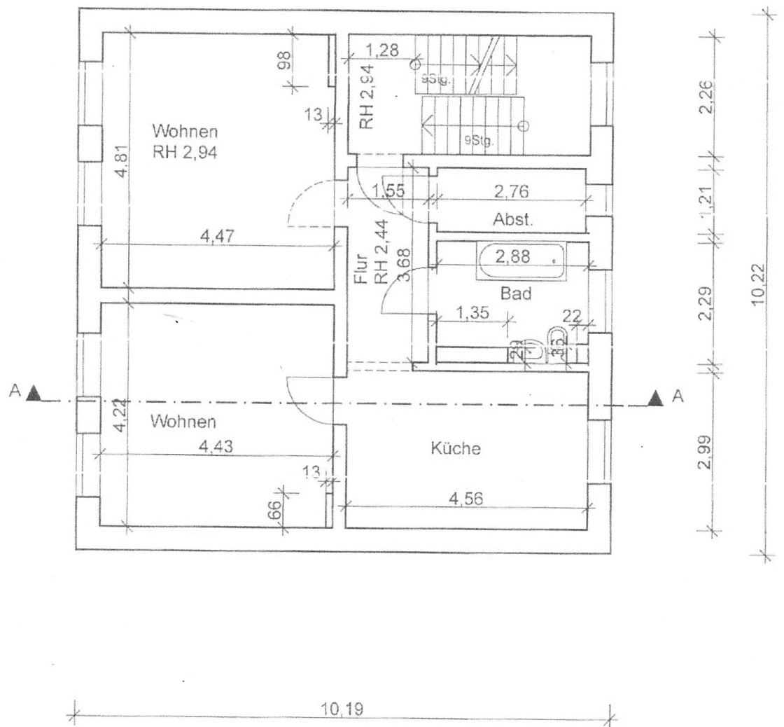
Grundriss Obergeschoss
