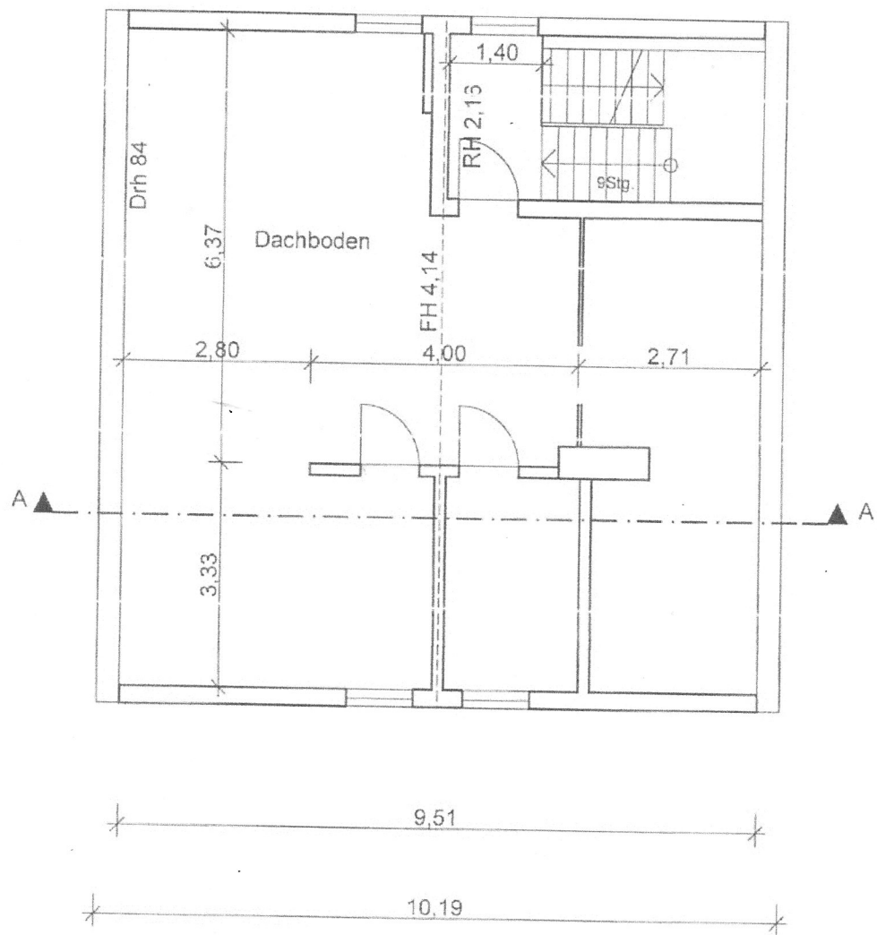
Grundriss Dachgeschoss
