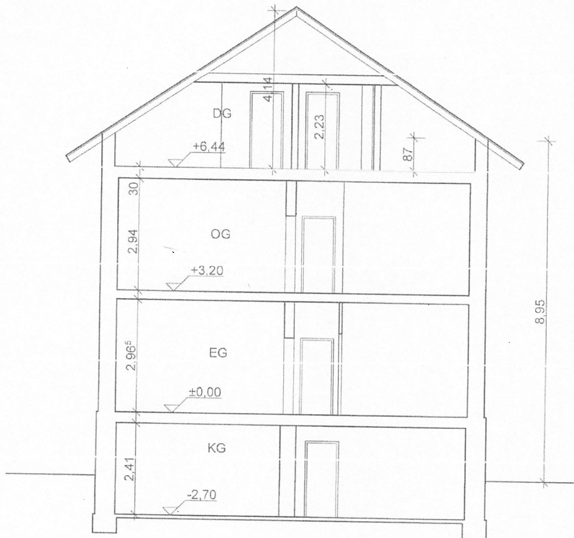
Schnitt A-A
