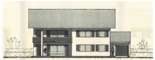
Süd-Ost-Ansicht
