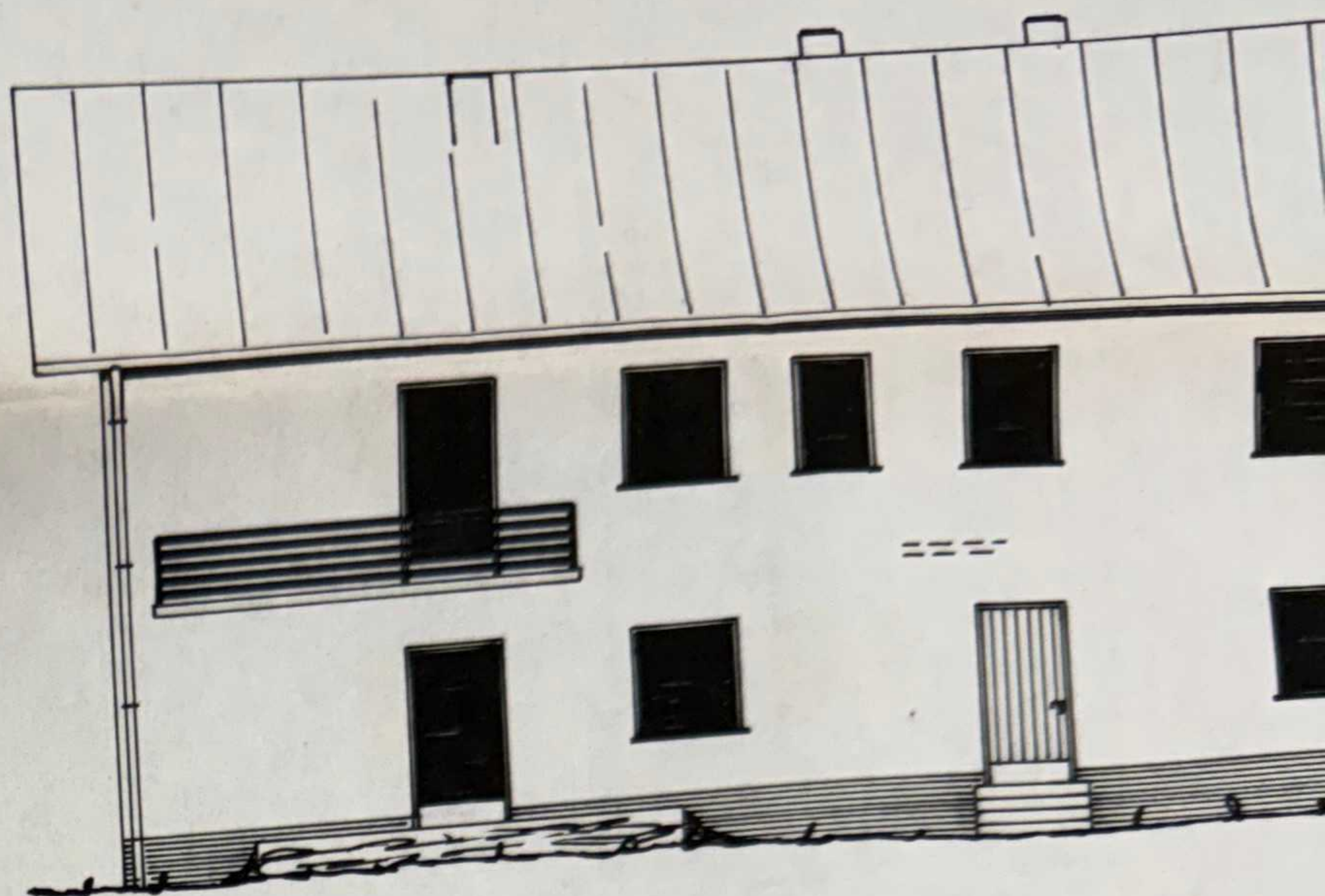
NORD - ANSICHT
