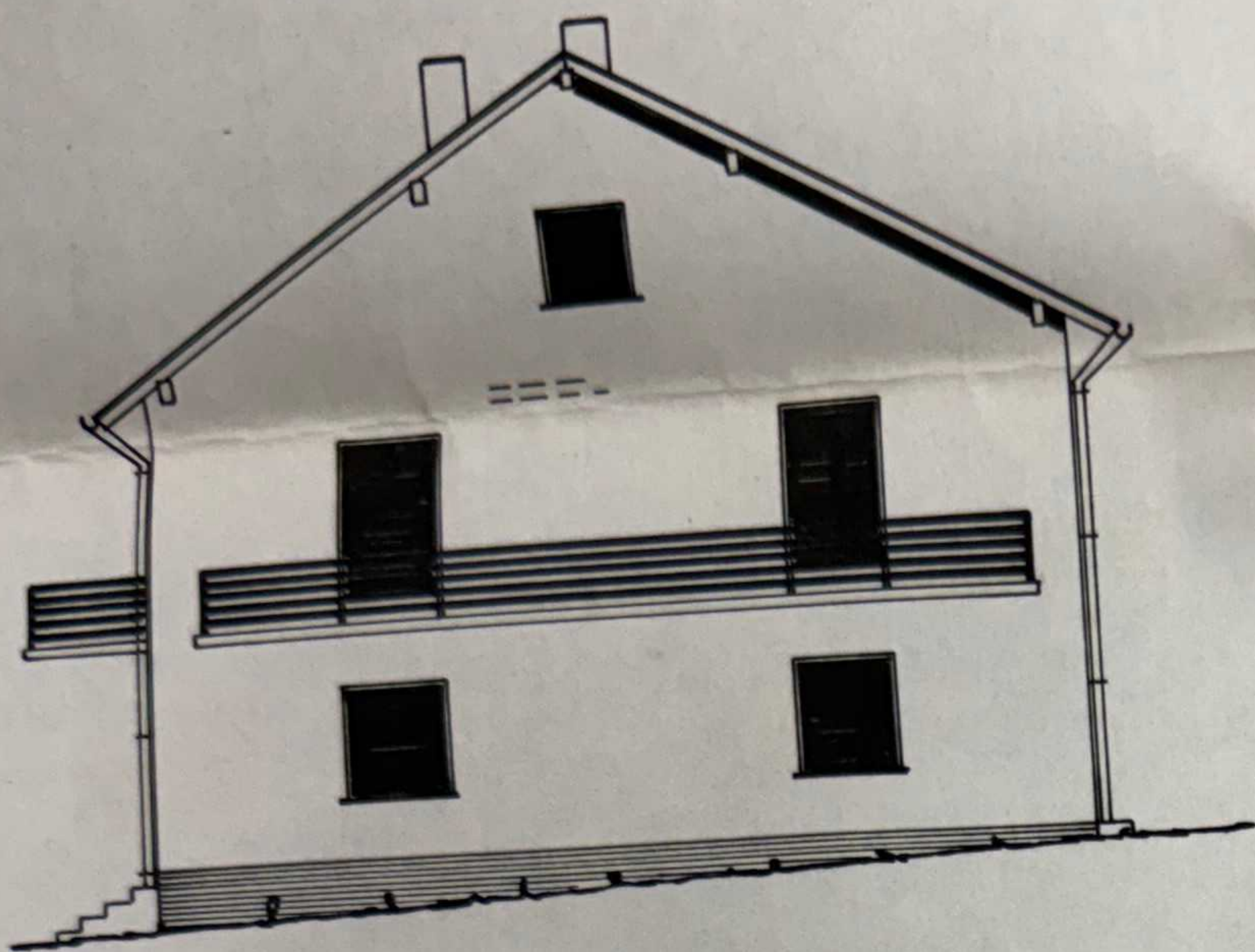
WEST - ANSICHT
