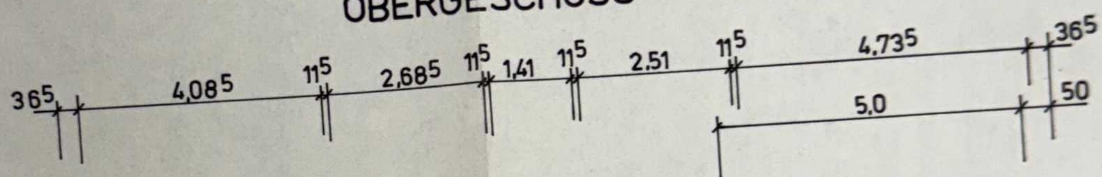
OBERGESCHOSS
