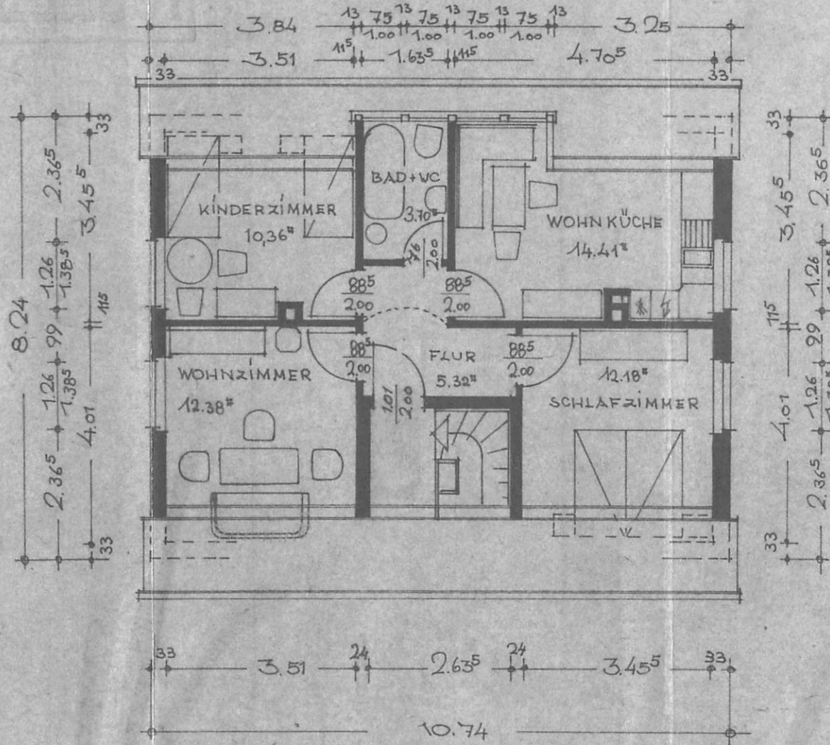
GRUNDRISS - DACHGESCHOSS
