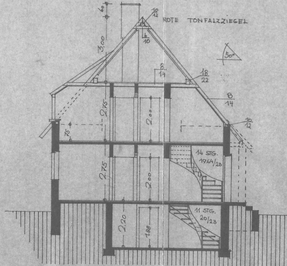
SCHNITT A-B
