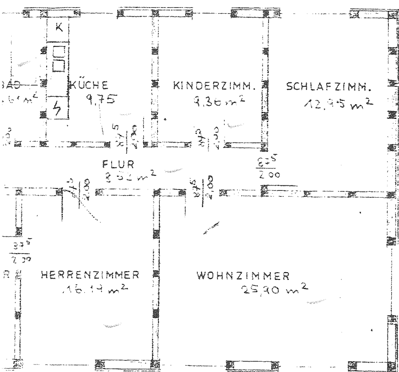
WOHNUNG II WOHNFLÄCHE 90.24 m²
