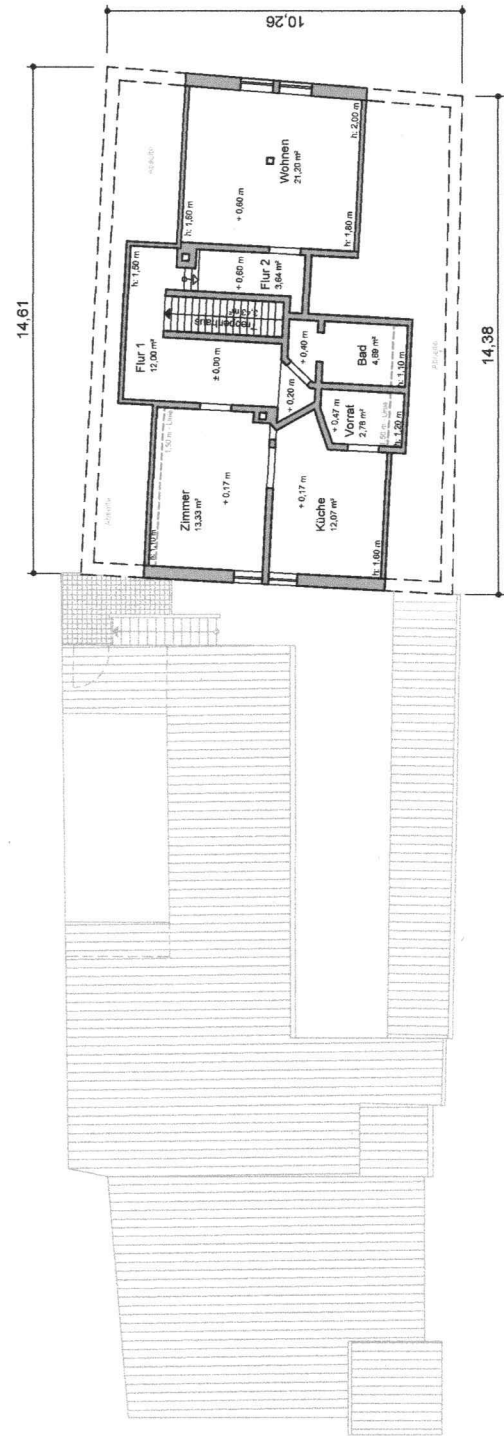
GRUNDRISSDG
