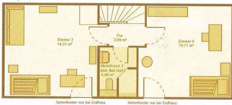
Dachgeschoss
