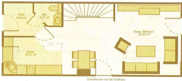
Erdgeschoss
