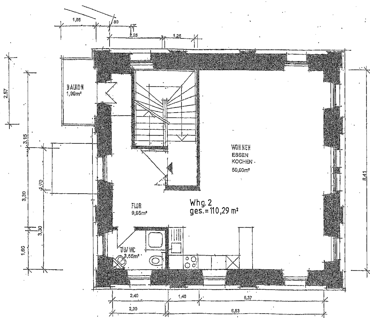
Obergeschoss M=1:100
