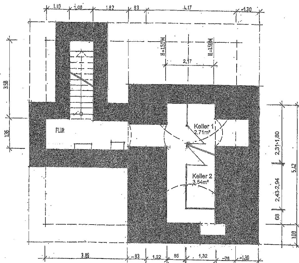
Kellergeschoss M=1:100
