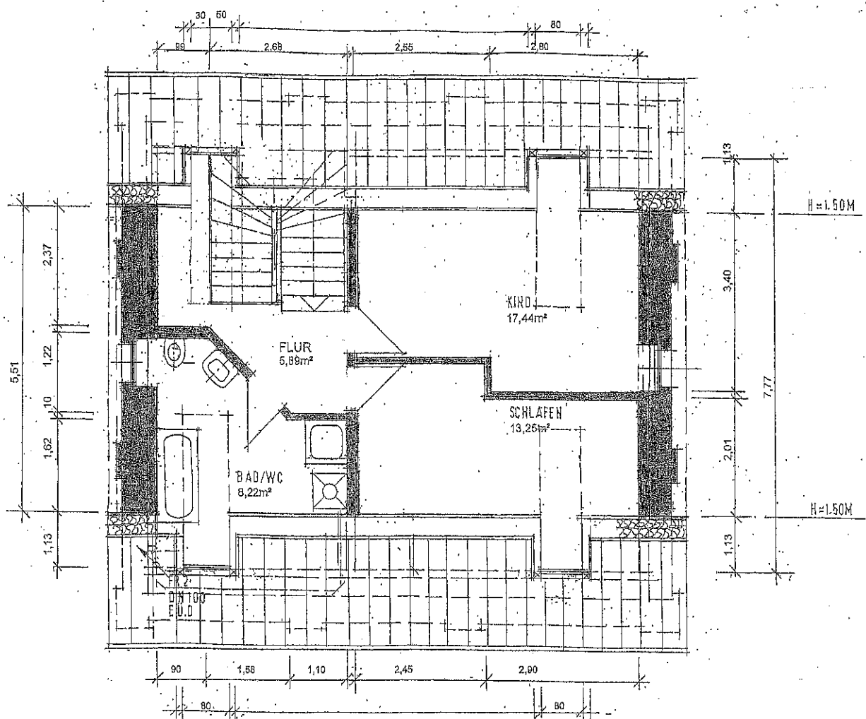
Dachgeschoss M=1:100
