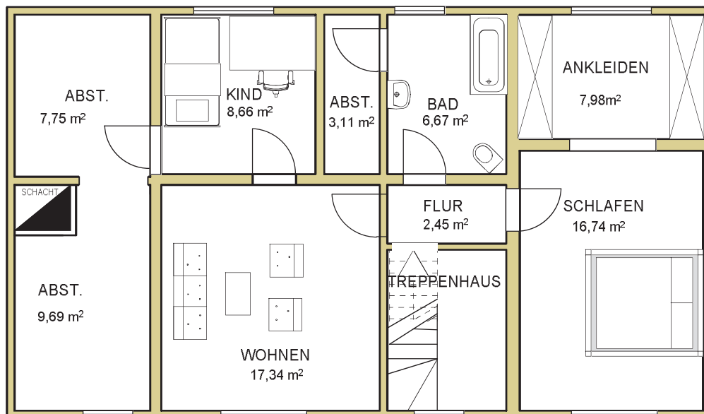
2. OBERGESCHOSS
