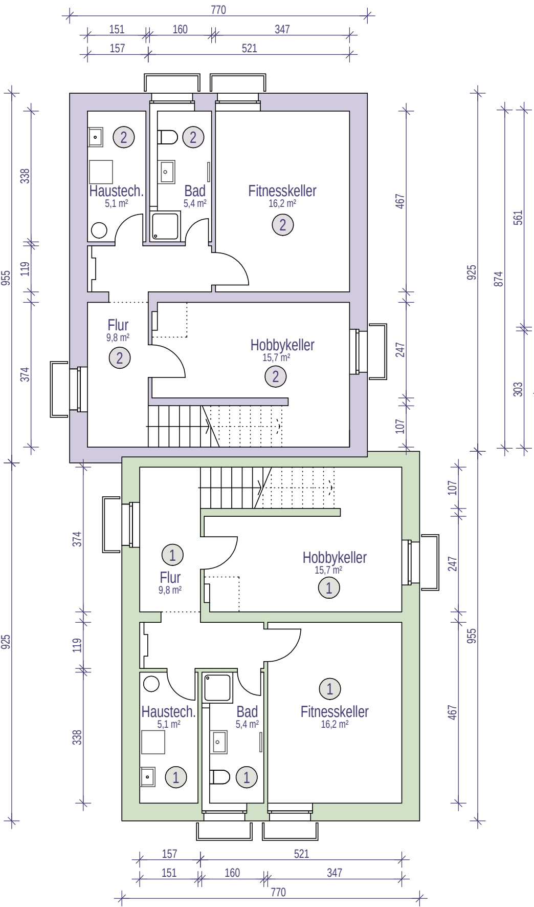
GRUNDRISS KELLER HAUS 1
