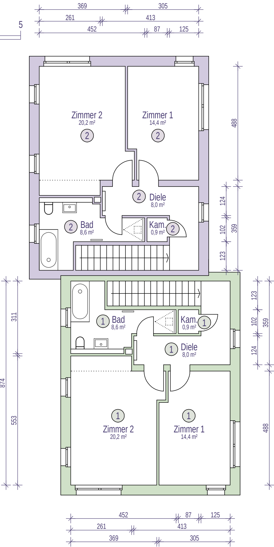
GRUNDRISS OBERGESCHOSS HAUS 1
