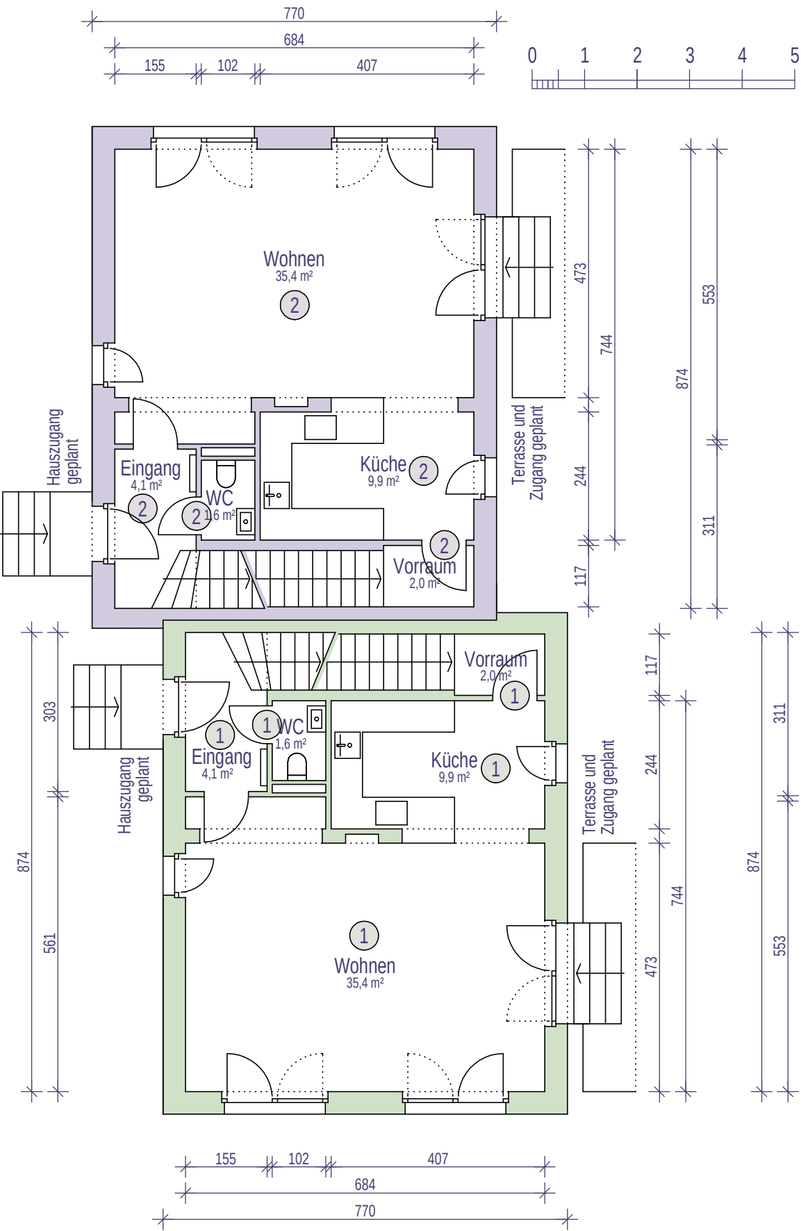
GRUNDRISS ERDGESCHOSS HAUS 1
