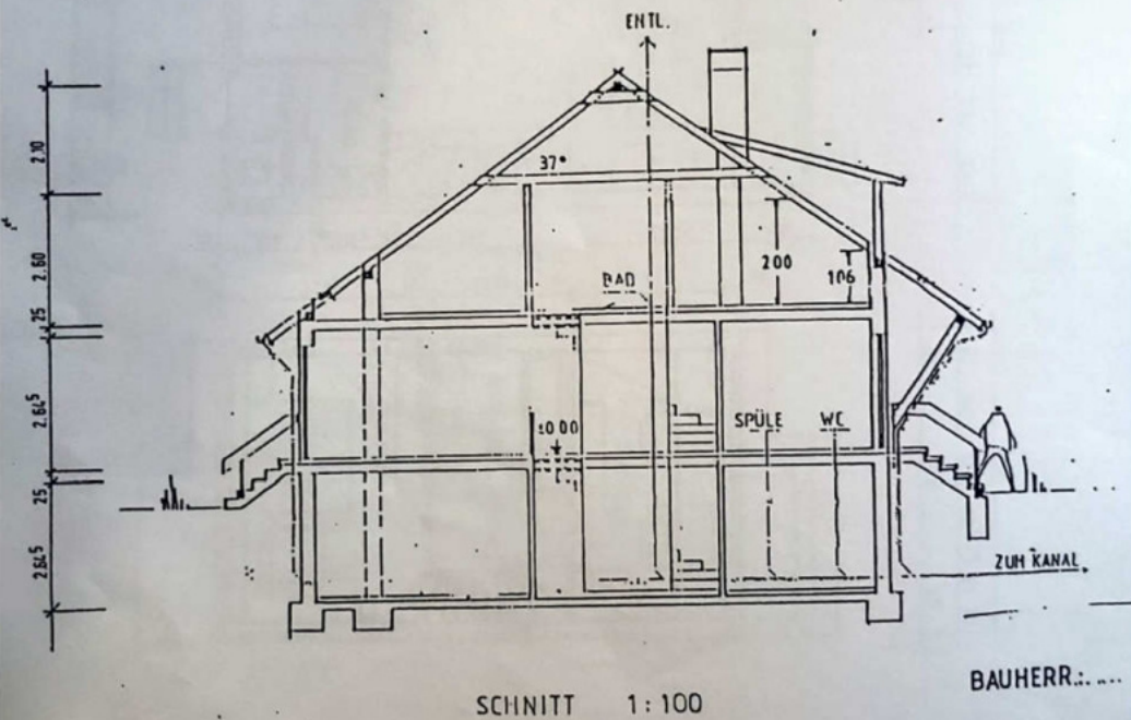
Abbildung 6: Schnitt
