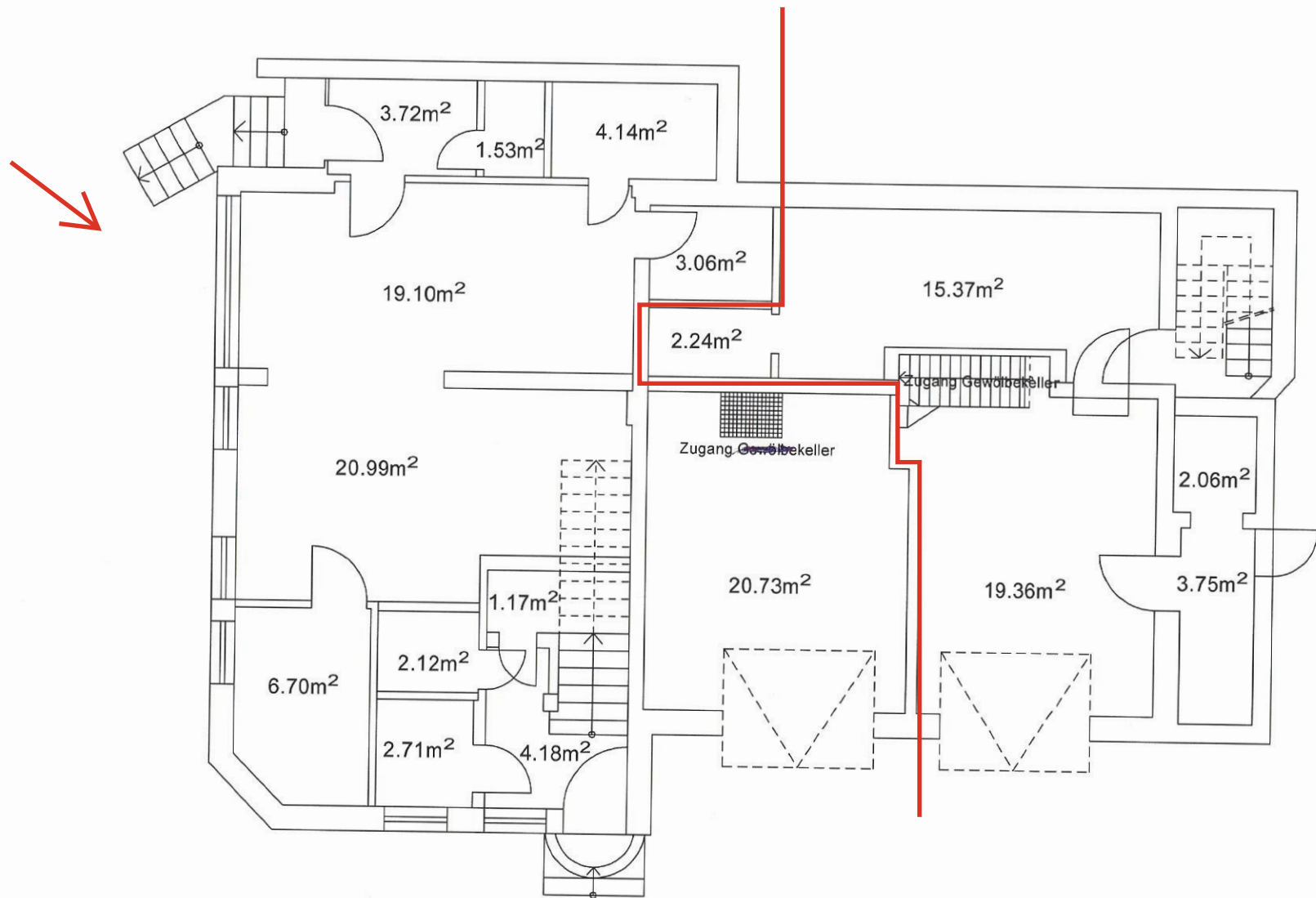
Kellergeschoss M 1:100
