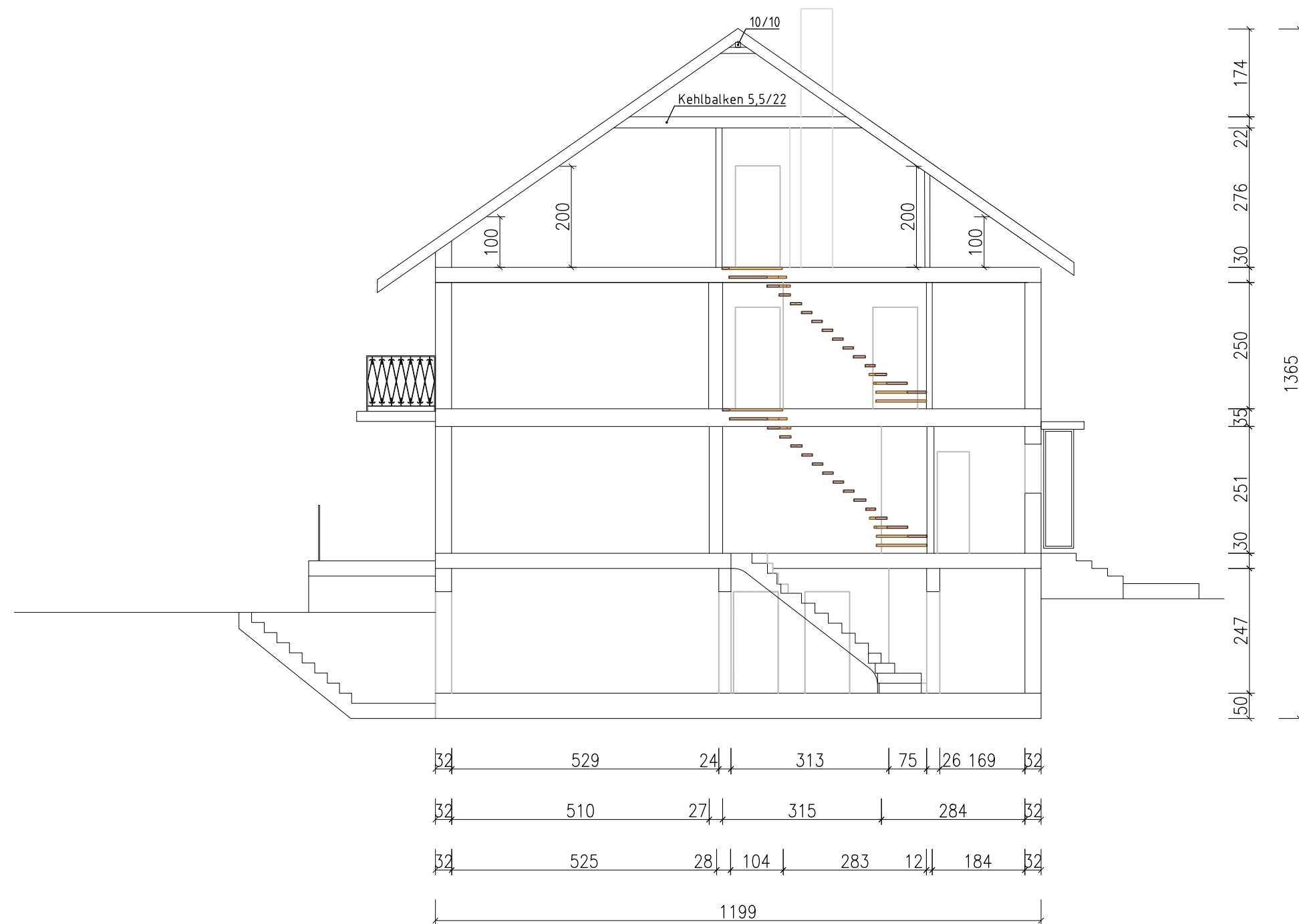
Schnitt A-A
