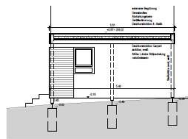
SCHNITT 4-4
