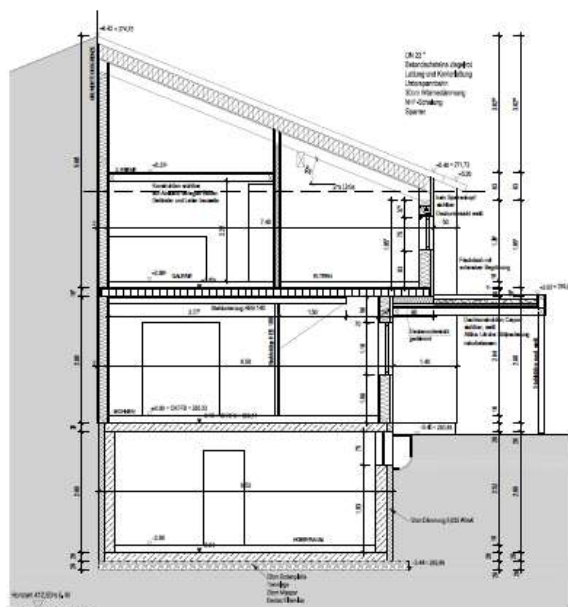
SCHN|TT 1-1
