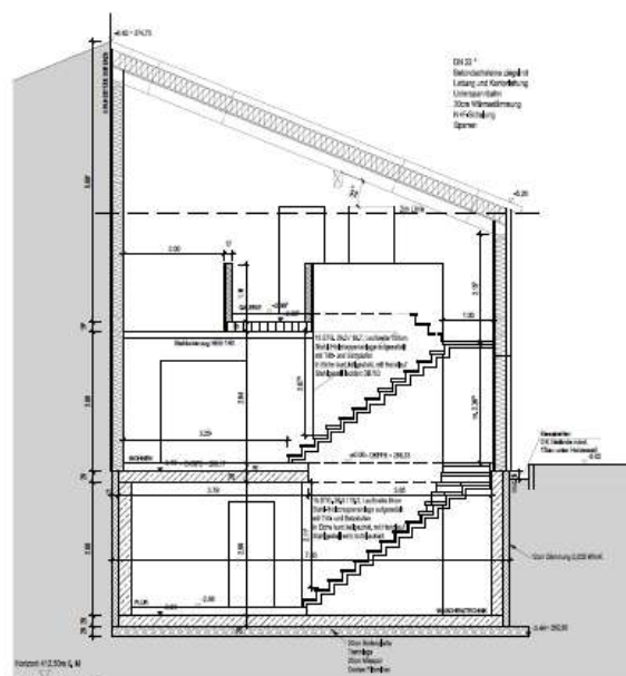
SCHNITT 2-2
