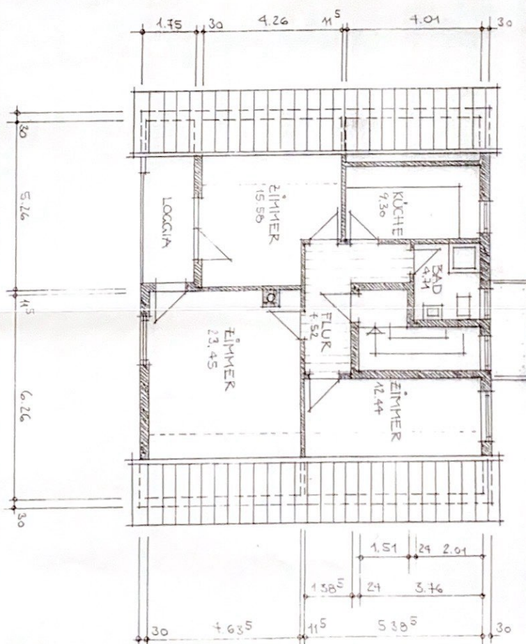
GRUNDRISS 1.100
