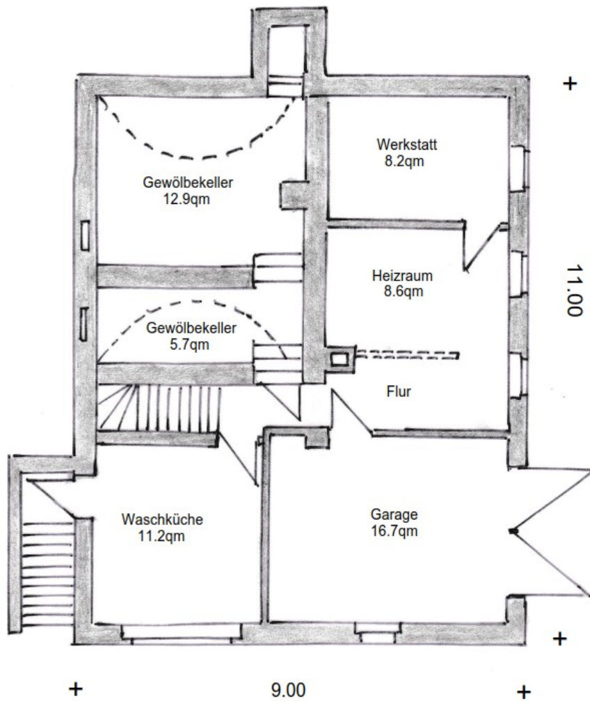
UNTERGESCHOSS
