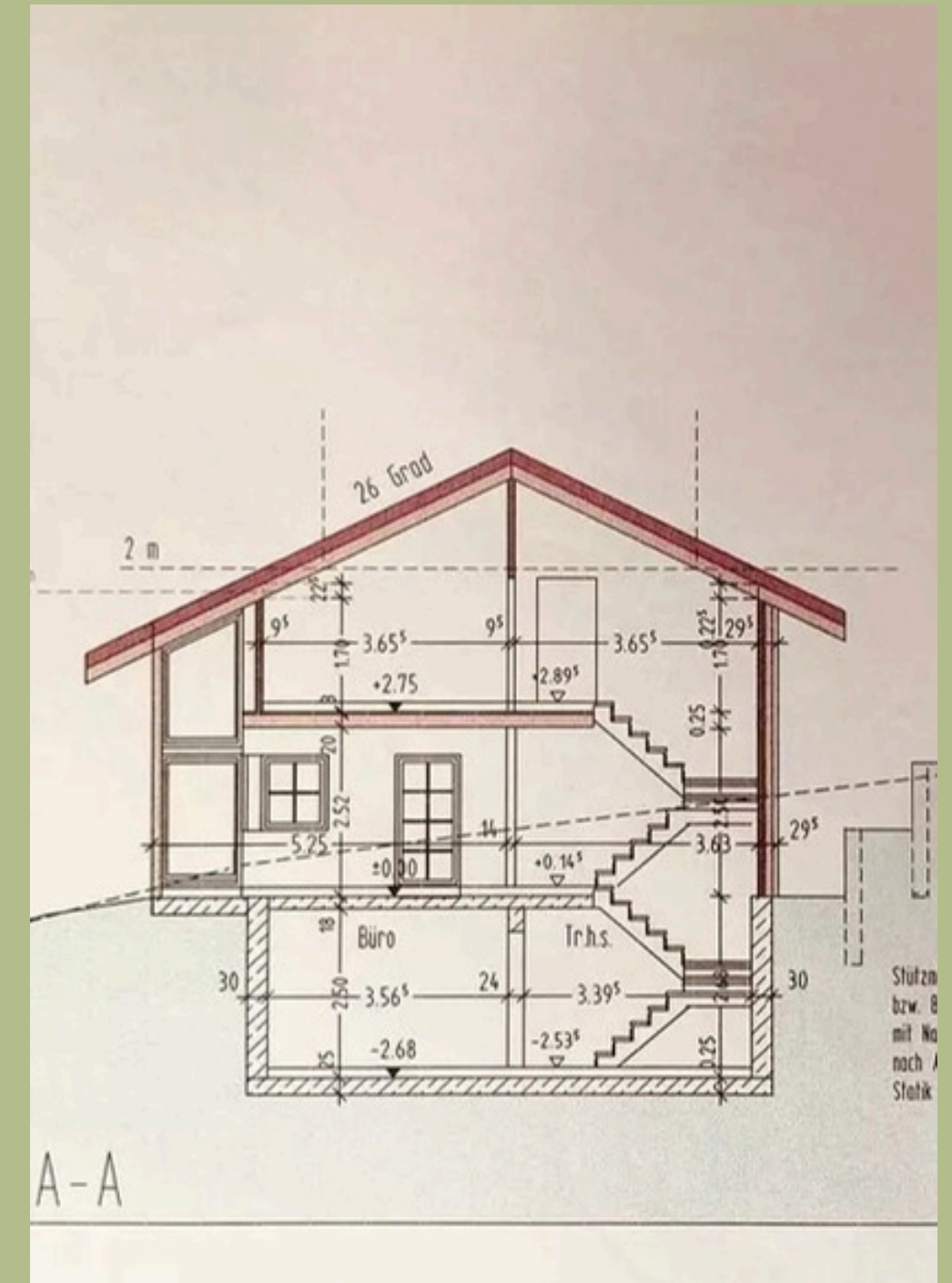
Schnitt
