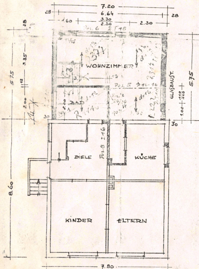
ERDGESCHOSS
