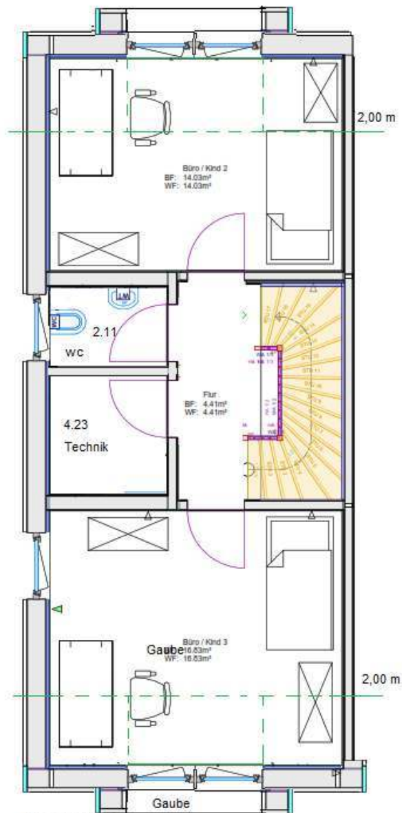
2 DACHGESCHOSS
