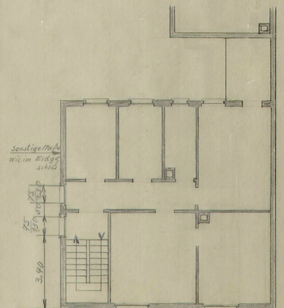
Grundriß: Obergerchoß
