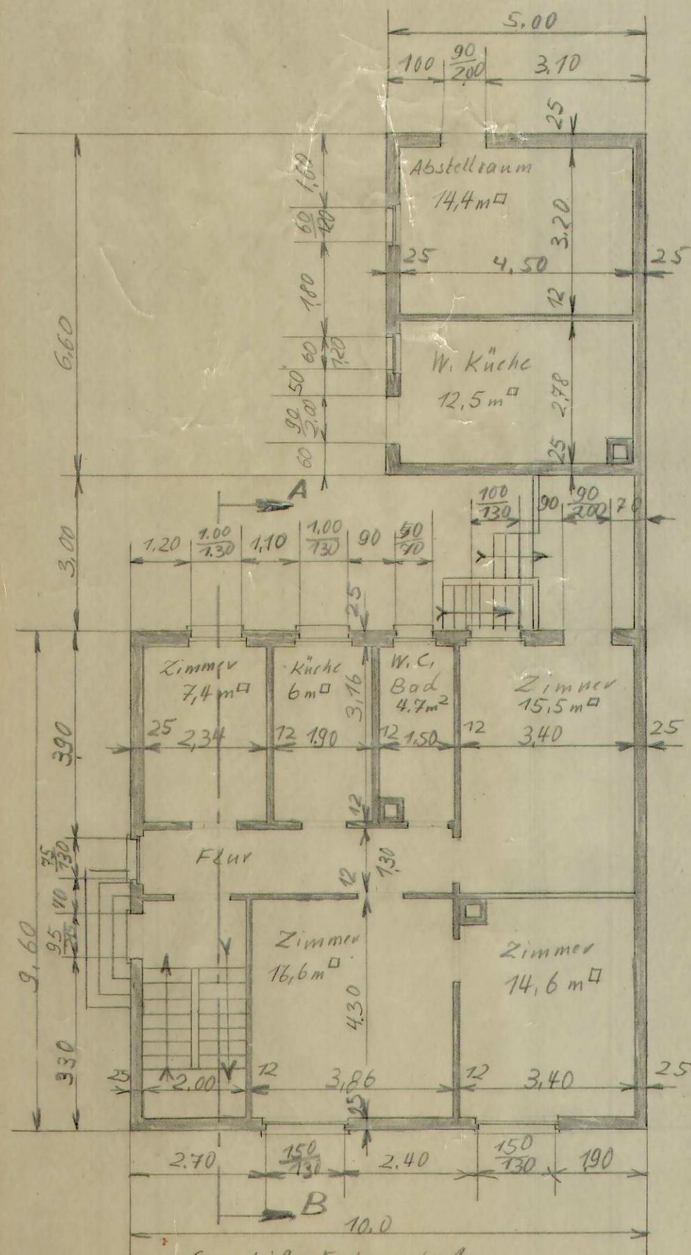
Grundriß: Erdgeschoss
