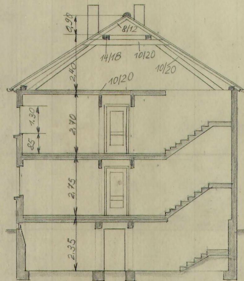
schnitt A-B
