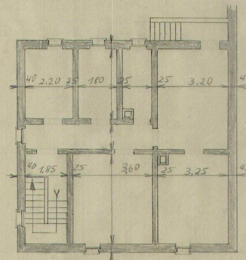
Grundriß: Kellergerchoß
