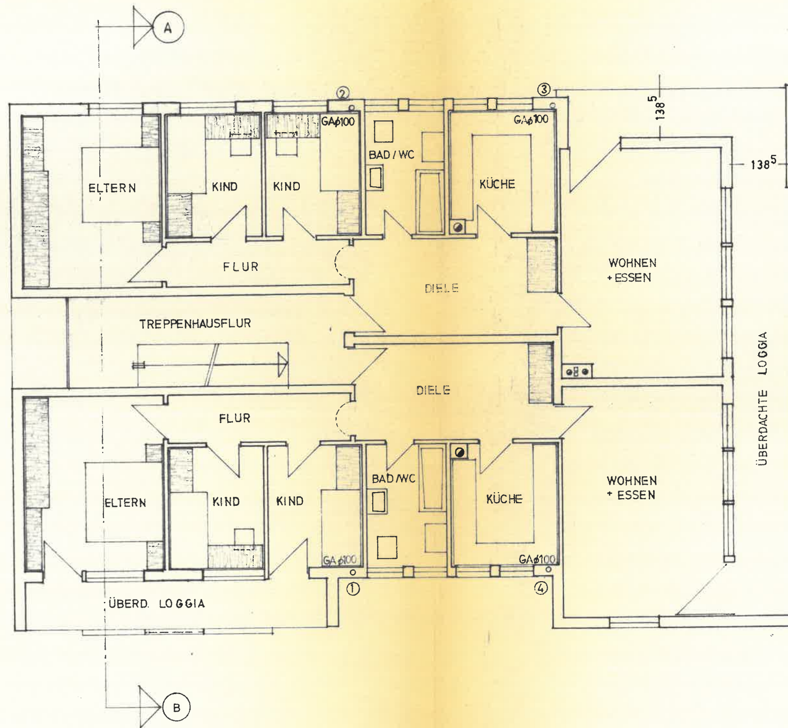
1. OBERGESCHOSS (MASSE WIE IM ERDGESCHOSS)
