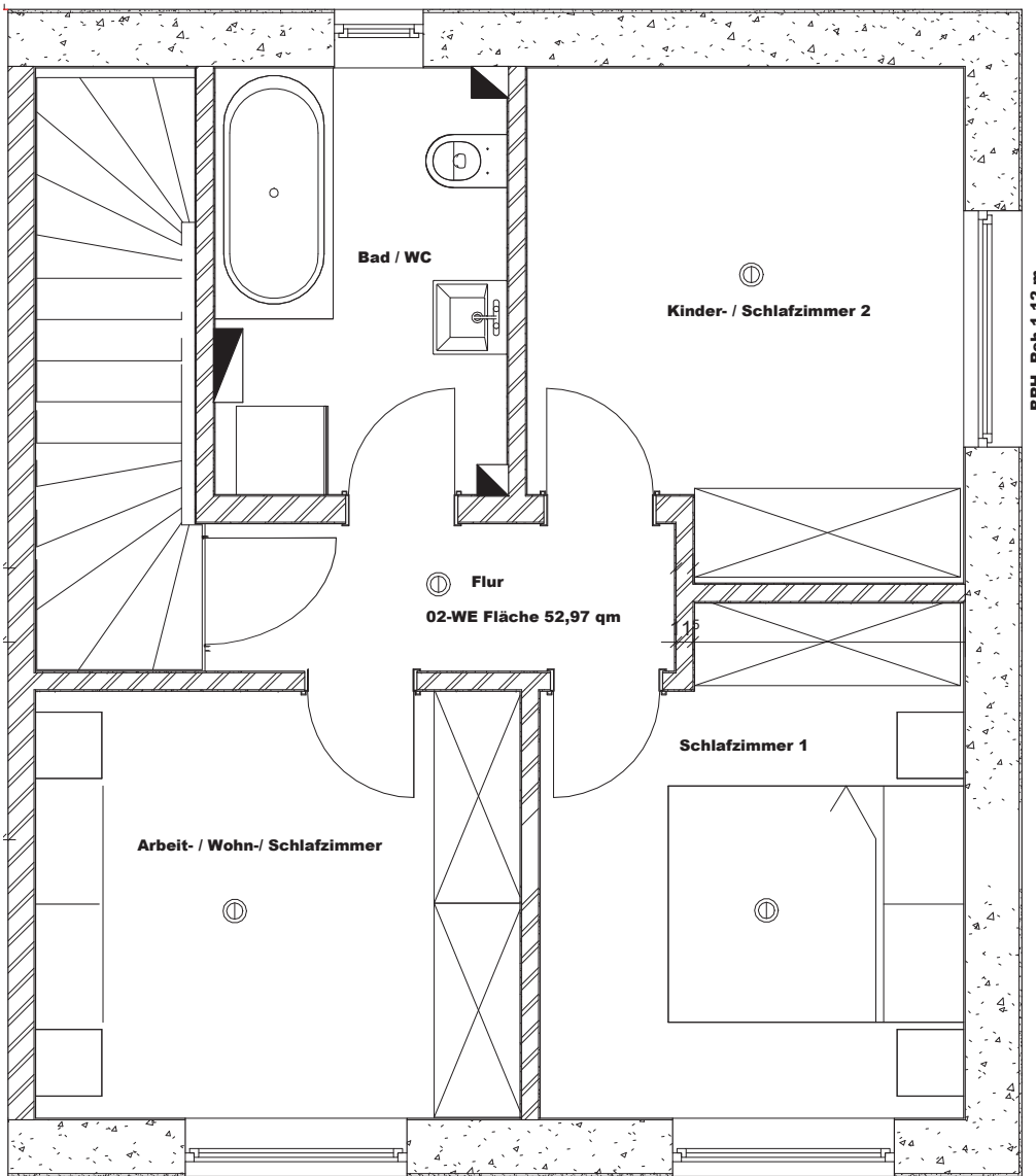
OBERGESCHOß LAYOUT
