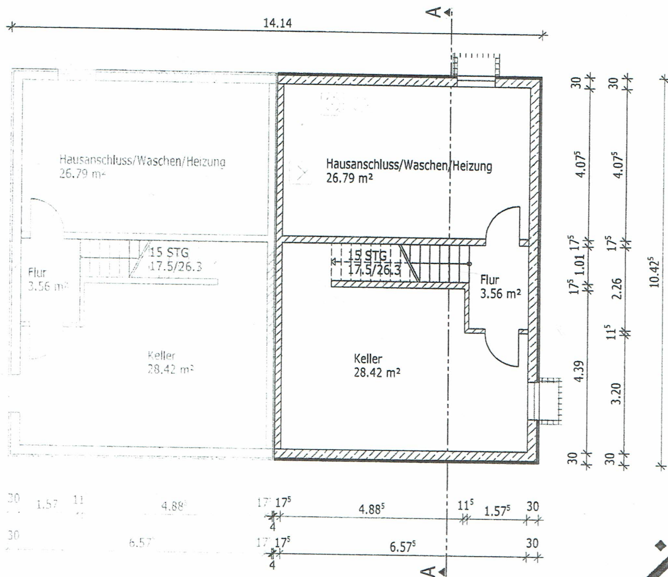
Grundriss Kellergeschoss
