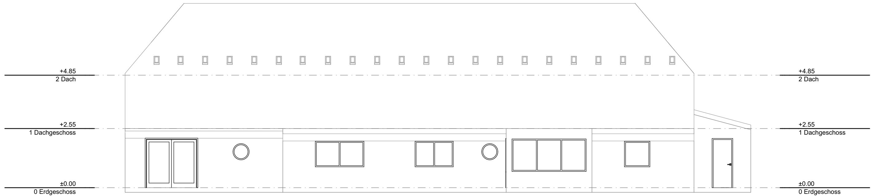
Südansicht 1:100
