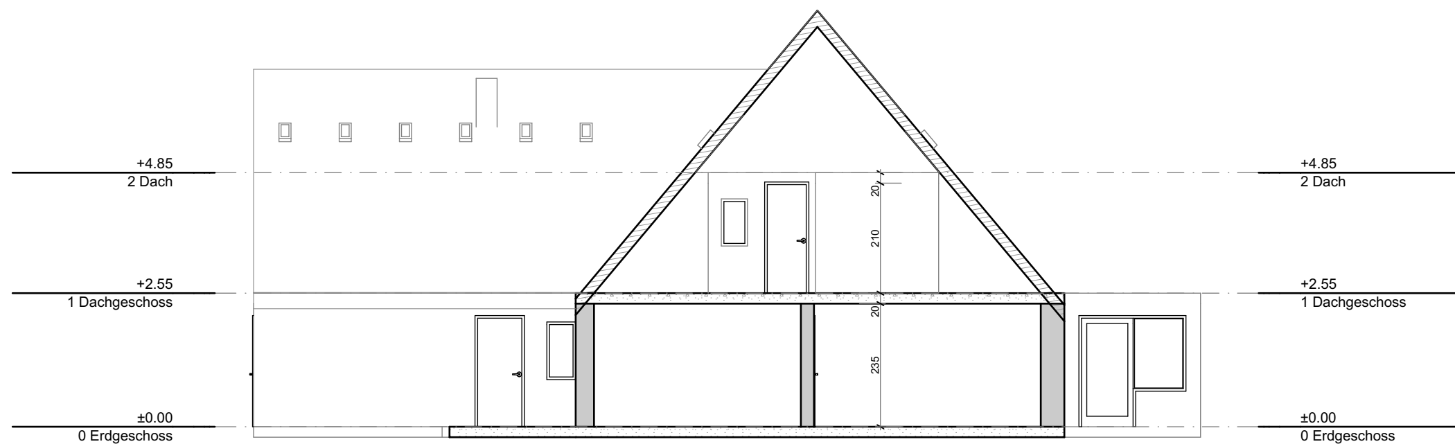
Schnitt 01 1:100
