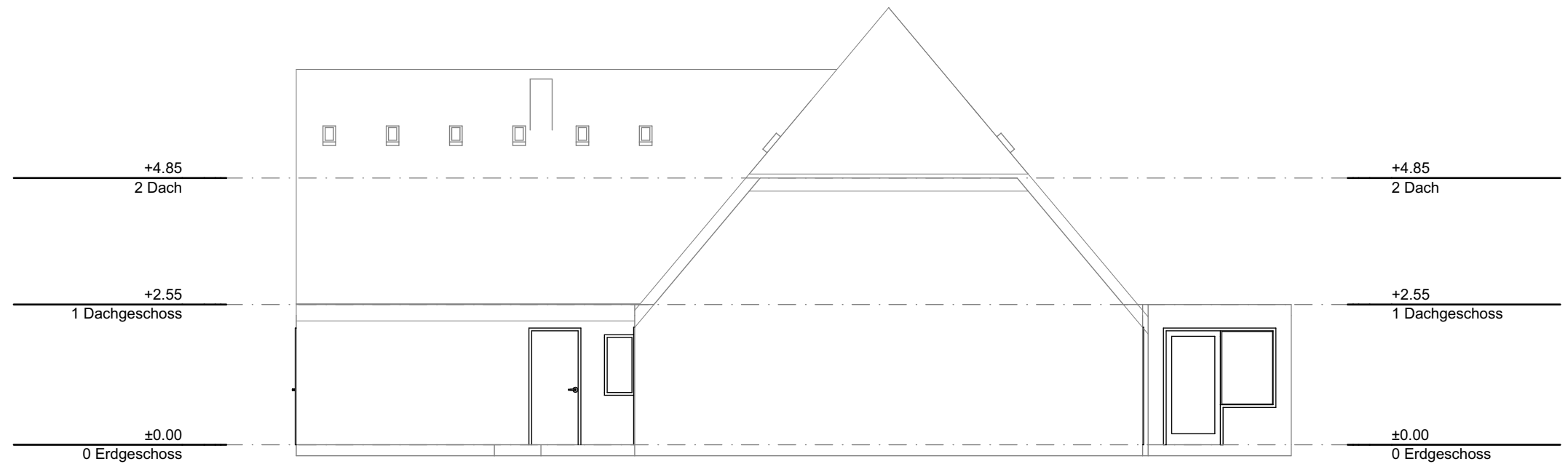
Westansicht 1:100
